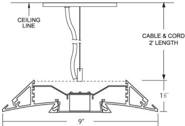
Cable Mount: Specify C code in catalog #
