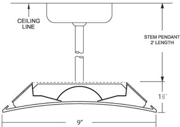
Swivel Stem Mount: Specify S code in catalog #
