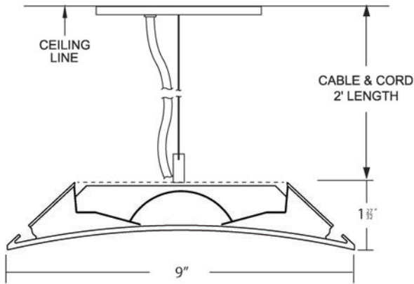
Cable Mount: Specify C code in catalog #
