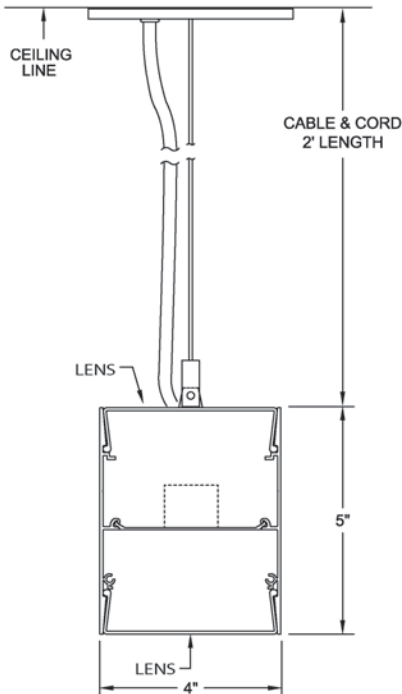
Cable Mount: Specify C code in catalog #
