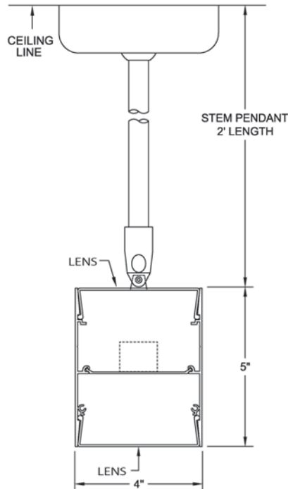
Swivel Stem Mount: Specify S code in catalog #
