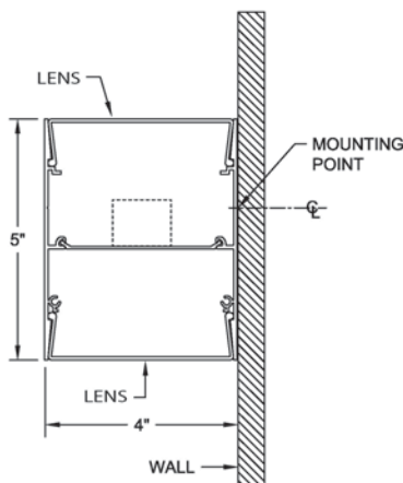
Wall Mount: Specify WM code in catalog #
