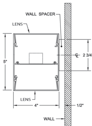
Wall Spacer Mount: Specify WSP code in catalog #
