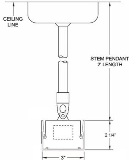
Swivel Stem Mount: Specify S code in catalog #
