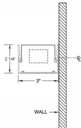
Wall Mount: Specify WM code in catalog #
