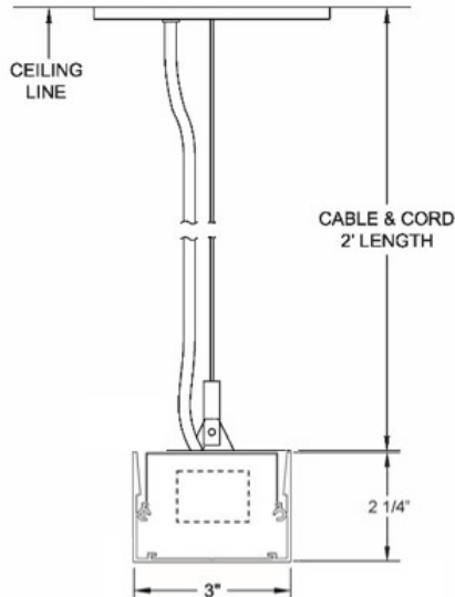
Cable Mount: Specify C code in catalog #
